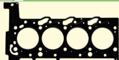
2601 086 Junta cabeçote Ranger/Transit 2.2/2.4 16V 11... Metalopak
