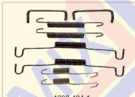
Patim sistema "varga" Corcel II/Belina II
