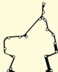
2601 057 Junta caixa da distribuição F-250/350/4000/Cargo 814 motor Cummins 4B/BTA 3.9L
