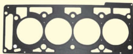
2601 052 2601 052 1 - Metal Junta cabeçote Escort 00.../Fiesta 99...Ecosport 03... 1.6 8V Zetec Rocam
