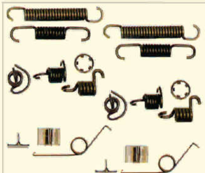
Patim sistema "bendix" Belina/Pampa 4 x 4 após 84(2rodas)
