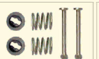
2600 259 Tras. Pampa 4x2 82/97 Del Rey 81/89 (39mm)
