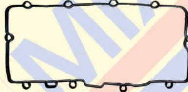
2601 065 Junta tpa. válvula Ranger 3.0 16V motor Power Stroke
