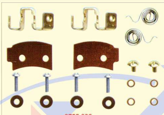
3755 006 Suporte escova (positivo) VW/CORCEL
