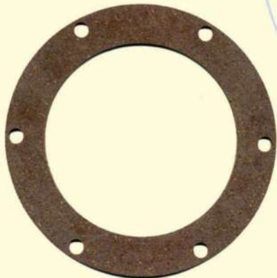
6566 105 Cubo carreta Krone (6 furos) Medida interna = 15,9cm Medida externa = 19,9cm Furos = 10mm, Largura = 2cm Espessura = 1.9cm
