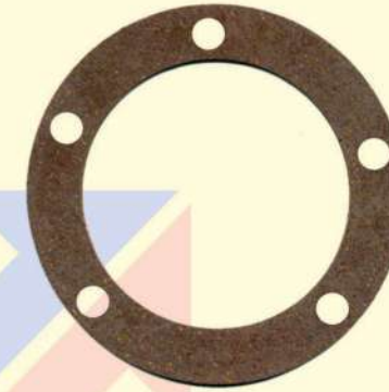
6566 103 Cubo carreta Randon(5 furos) Medida interna = 15,9cm Medida externa = 20,1cm Furos = 10mm, Largura = 2.2cm Espessura = 2mm
