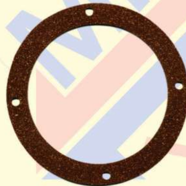
6566 106 Cubo carreta Master (4 furos) Medida interna = 14cm Medida externa = 18,4cm Furos = 8mm, Largura = 2cm Espessura = 2mm
