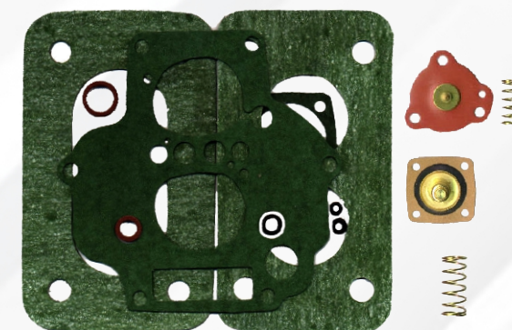
3566 505 - Jogo de Junta Corcel/Belina/Escort/Scala C/ Motor CHT 1.6 07/83... Carb. 460 Alc.
