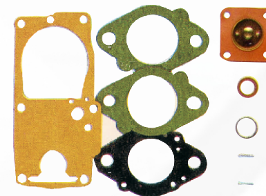
3566 525 - Jogo de Juntas CHEVETTE/MARAJÓ 1.4 85...86 Carb. 118 gas.
