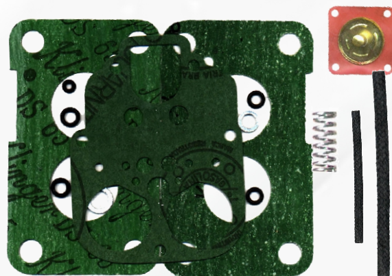
3566 506 - Jogo de Junta Corcel/Passat/Gol/Voyage/Parati 1.6 (Refrig. Água)/Chevette 1.4 e 1.6 Carb. 450 (Mini Progressivo) Alc./Gas.
