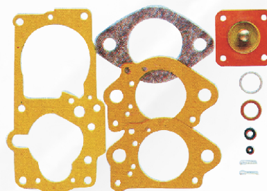
3566 531 - Jogo de Juntas CHEVETTE 1.6 84... Carb. 040 álc.
