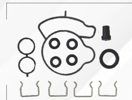
3566 600 Ford Ka-Fiesta-Courier 1.4 MPFI c/ motor Zetec - 16V
