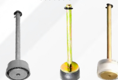
4008 514 CHEVETTE/MARAJÓ motor 1.4 Gasolina 400.770.02 Carb. 228
