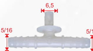
4008 300 476 Adaptador emenda mang. combustível em T 5/16x5/16x6,5
