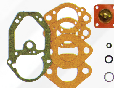
3566 070 - Reparo completo 3566 515 - Jogo de juntas FIAT 1050/1300 ...82 Carb. 070 álc./gas.
