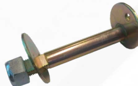
6200 301 2 Parafuso reg. cambagem Toyota Hilux 97...04 M16x1,5x115
