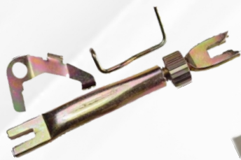
Regulador freio sist. varga (01 roda) Renault Clio 6200 607 - tras./dir. 6200 607 1 - tras./esq.
