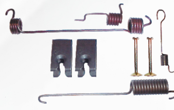
4600 134 Reparo sapata freio tras. esq/dir Celta/Prisma - 31mm
