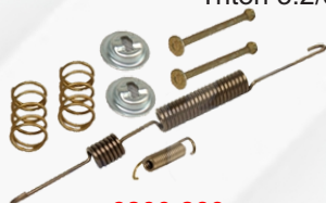
6200 289 Reparo da sapata freio (p/ 1 roda) tras. dir./esq. Toyota Hilux ...04
