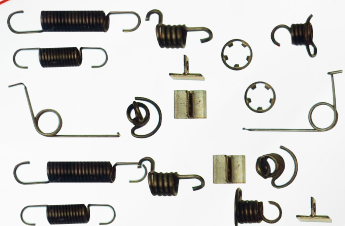
4600 186 1 Reparo patim (Bendix) Chevette/Marajó/Chevy 500 ...86
