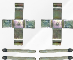
1600 391 Reparo freio disco diant. (p/ 2 rodas) Sist. A.Teves - Kombi 1600 82...
